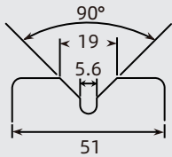
V槽铸铁轮宽深尺寸
